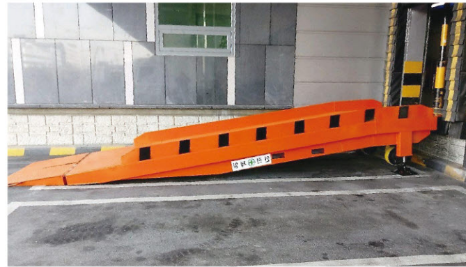
이동식 DECK RAMP (Mobile Type Deck Ramp)
